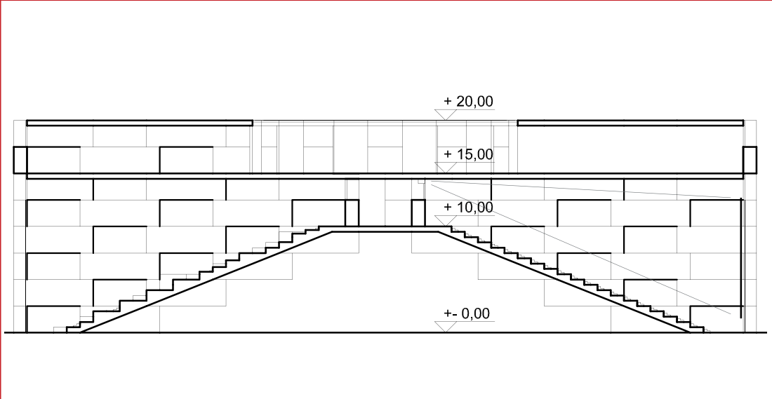
Längsschnitt M1/500
