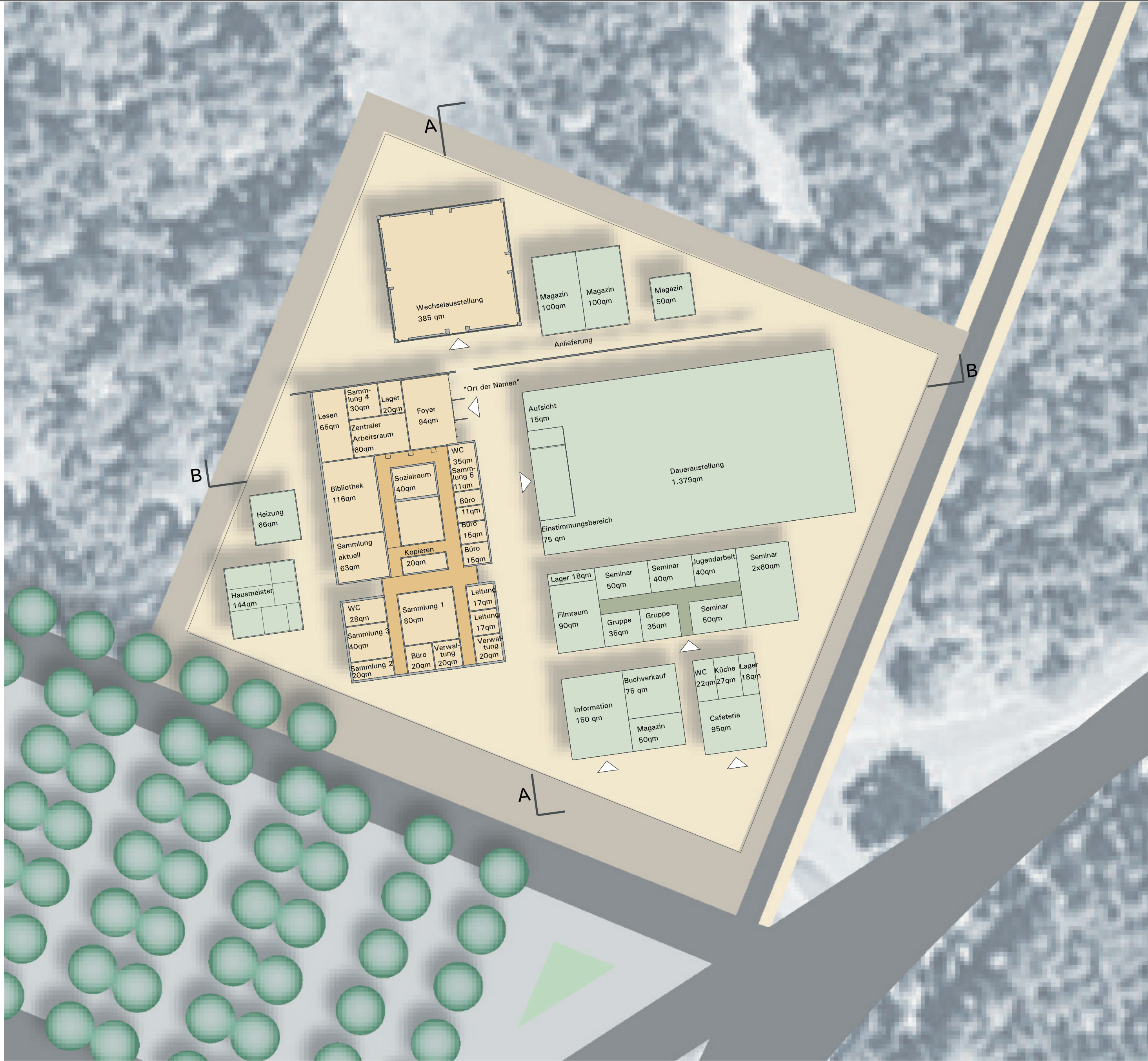
Grundriss M1/500
